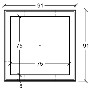
PLANTA ARQUETA
