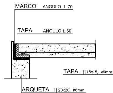
DETALLE ESCALA 1/10
