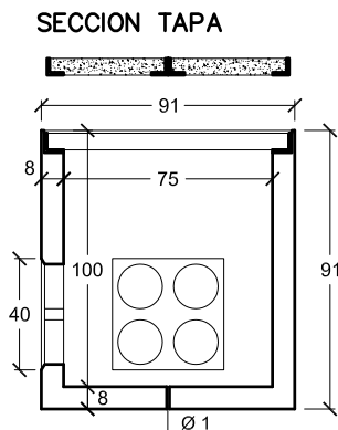
SECCION
