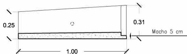
SECCIÓN a-a'
