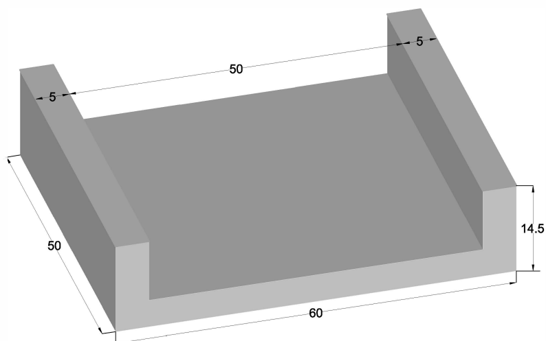
VISTA A
