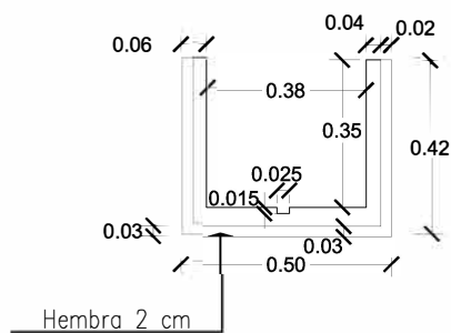
VISTA HEMBRA
