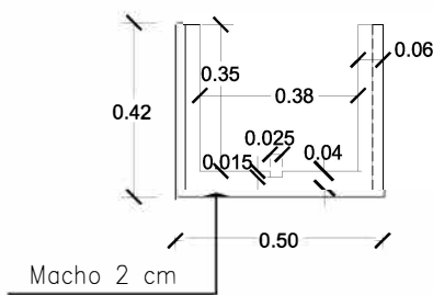
VISTA MACHO
