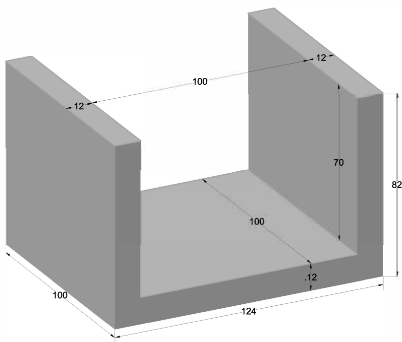
PERSPECTIVA cotas en cm.
