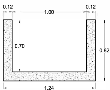
SECCION a-a'
