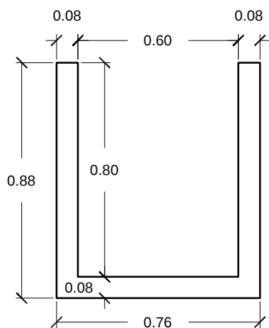
VISTA A
