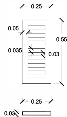
REJA DE HORMIGÓN armado de Ø4 mm.
