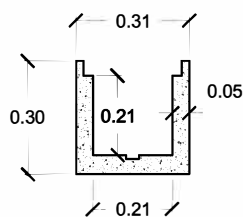
SECCIÓN a-a'
