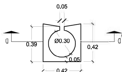
VISTA HEMBRA
