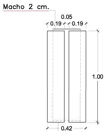
Hembra 2 cm.
