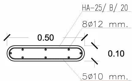
SECCIÓN a-a'
