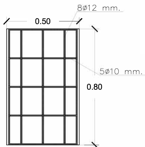
SECCIÓN b-b'
