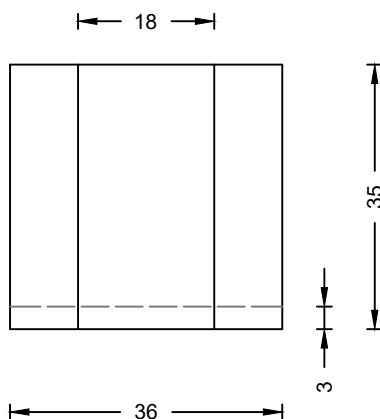
ALZADO (CON FONDO)
